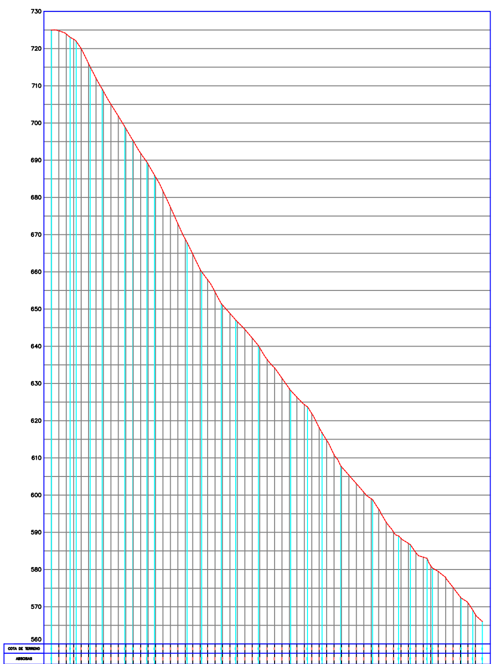
PERFILES Escala H= 1:10000 V= 1:20000
